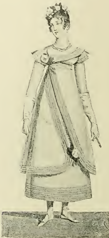
Fig. 545 Mode de 1819.
